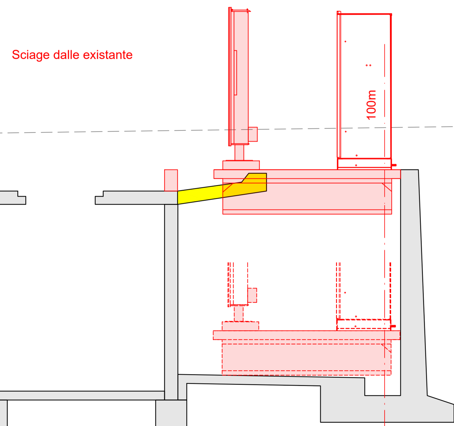
Détail chambre de cibles - 1:20 - structure béton armé -
